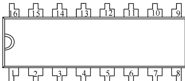
图 2 KA7500B 管脚
